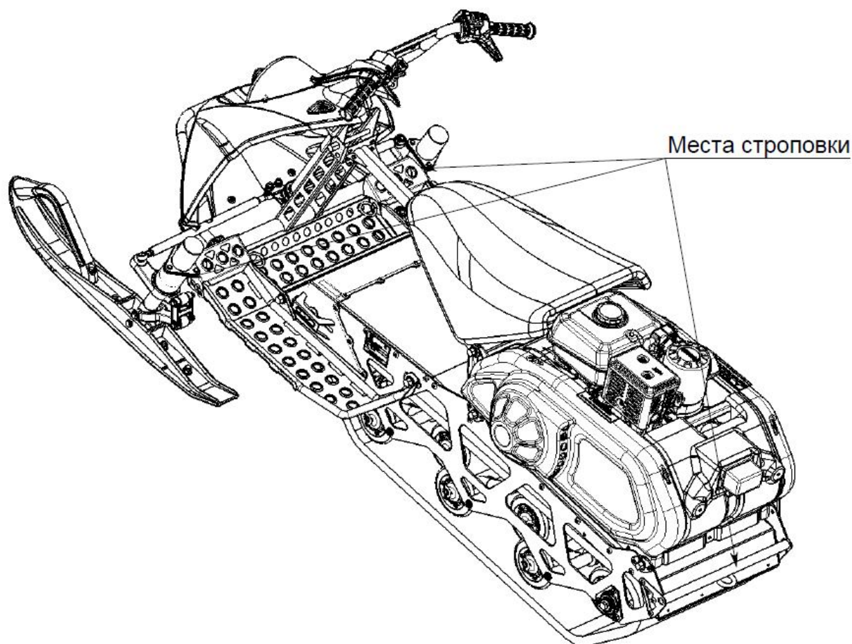
Рисунок 8 – Строповка средства малой механизации
