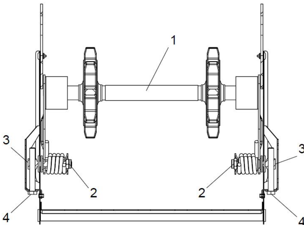
1 – вал направляющий; 2 – гайка; 3 – ось балансира; 4 – болт
