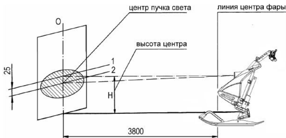
Рисунок 15 – Регулировка фары
