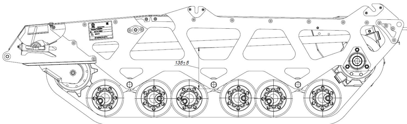
Рисунок 12 – Проверка натяжения гусеницы
