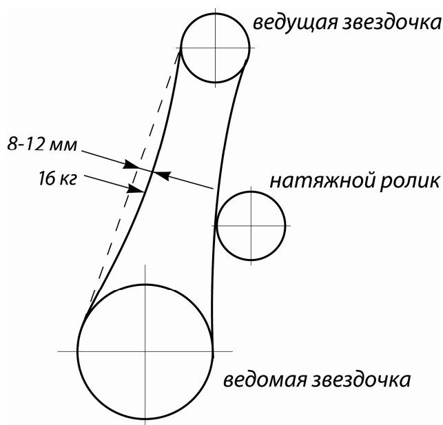
Рисунок 11 - Схема проверки натяжения цепи от промежуточного вала к приводному валу двигателя
