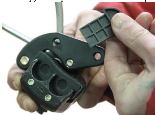
3.6.2. Из механизма переднего дискового тормоза вытащите транспортировочную заглушку, препятствующую сведению колодок.
