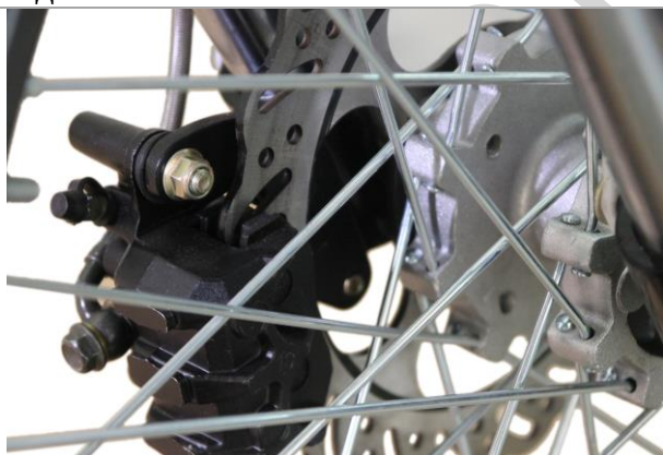
3.6.4. Установите тормозной суппорт на тормозной диск.
